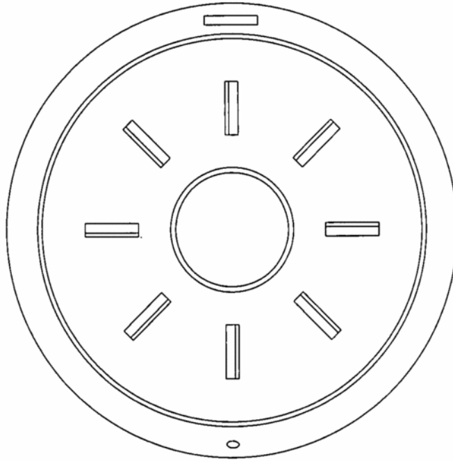
右側視圖
